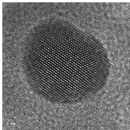
Obrázek 1. Nanočástice stříbra na silikátové částici. Připraveno jako přísada do antibakteriální nátěrové hmoty. Snímky pro nás připravila spolupracující laboratoř na TU Freiburg.
