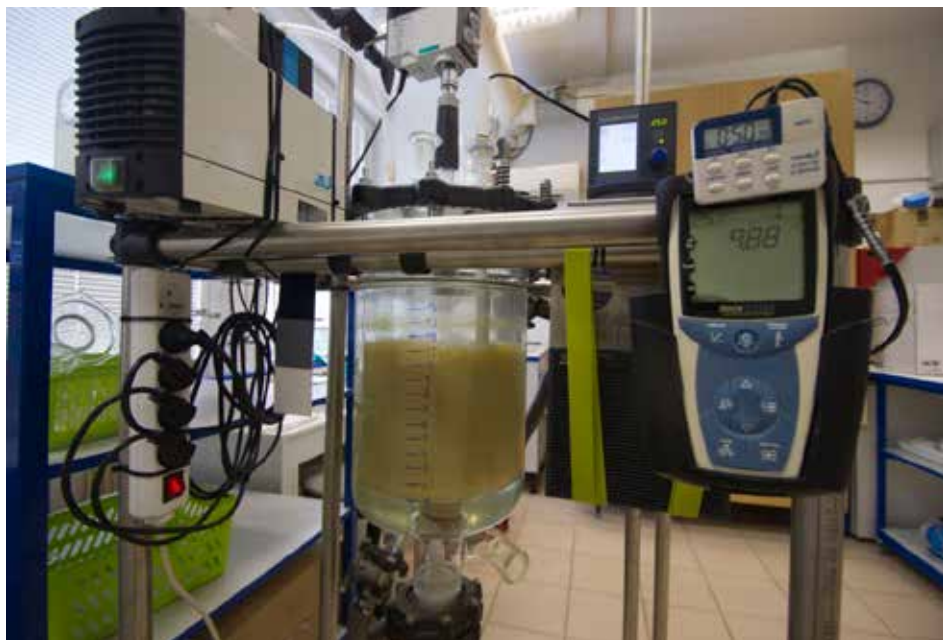
Obrázek 2: Reaktor pro přípravu nanočástic oxidů kovů v koloidních roztocích na Fakultě životního prostředí UJEP.
